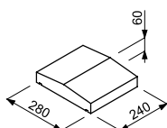
CBG daszek murkowy gładki dwuspadowy
