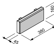
GP błoczek murkowy łupany jednostronnie
