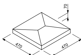
CSDR daszek słupkowy gładki czterospadowy
