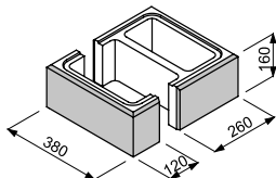
GUD+GAD błoczek słupkowy łupany czterostronnie
