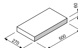
CPGM daszek murkowy łupany dwustronnie
