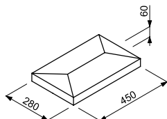
CSBNR daszek słupkowy gładki czterospadowy
