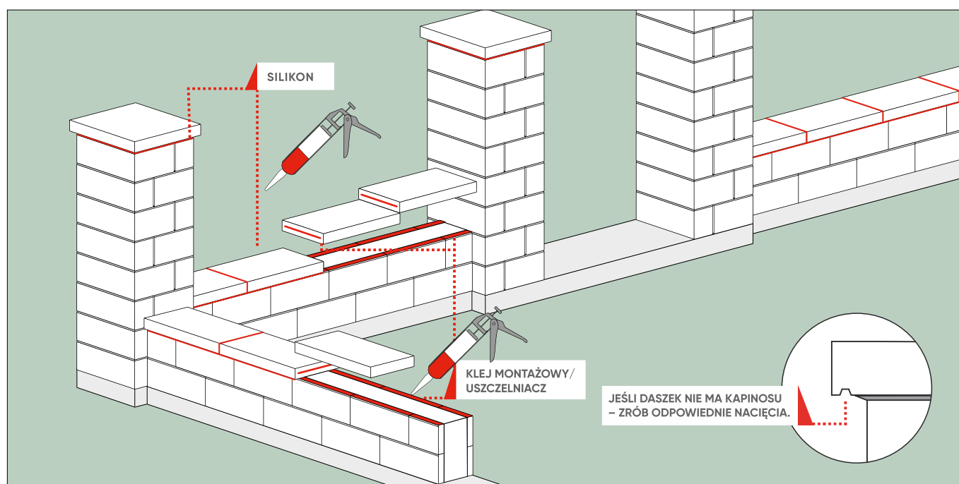
montaż daszków
