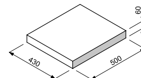
CPGMD daszek murkowy łupany dwustronnie
