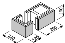
GU+GA błoczek słupkowy łupany czterostronnie
