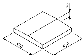
CPDD daszek murkowy gładki dwuspadowy
