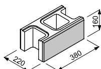
GM błoczek murkowy łupany dwustronnie
