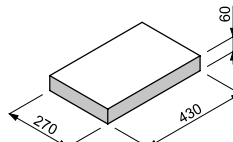
CPGS daszek słupkowy łupany czterostronnie
