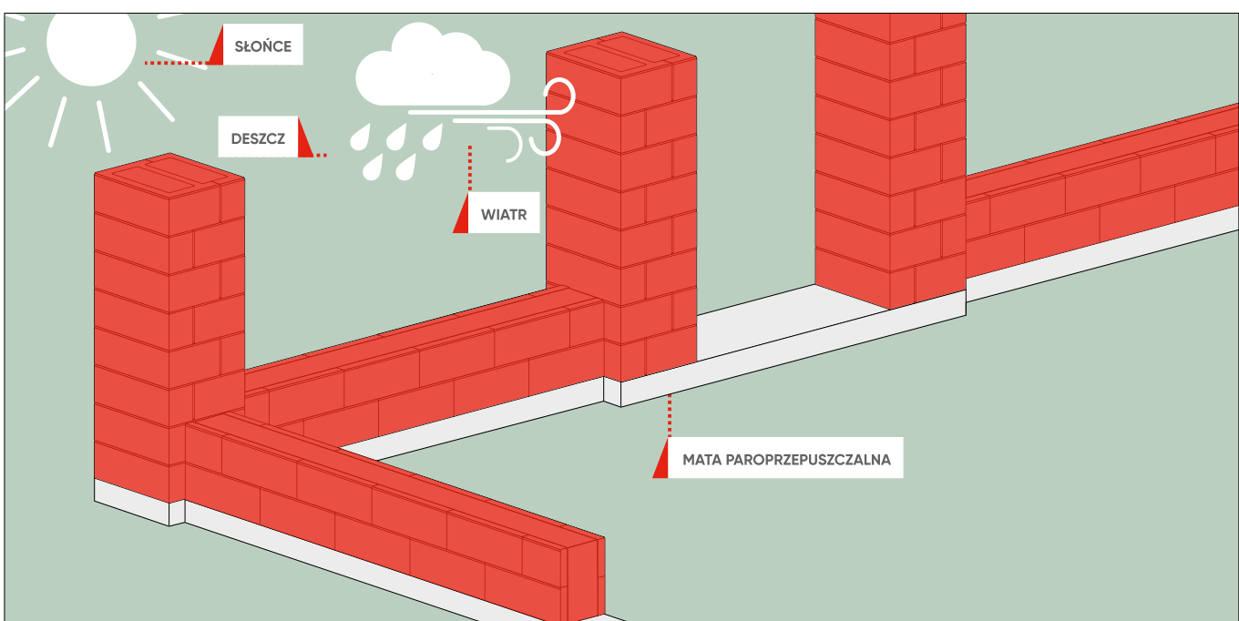
pielęgnacja betonu
