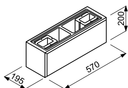
RVE19, RVEM19 błoczek słupkowy / murkowy
