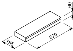
CRVE19, CRVEM19 daszek słupkowy / murkowy
