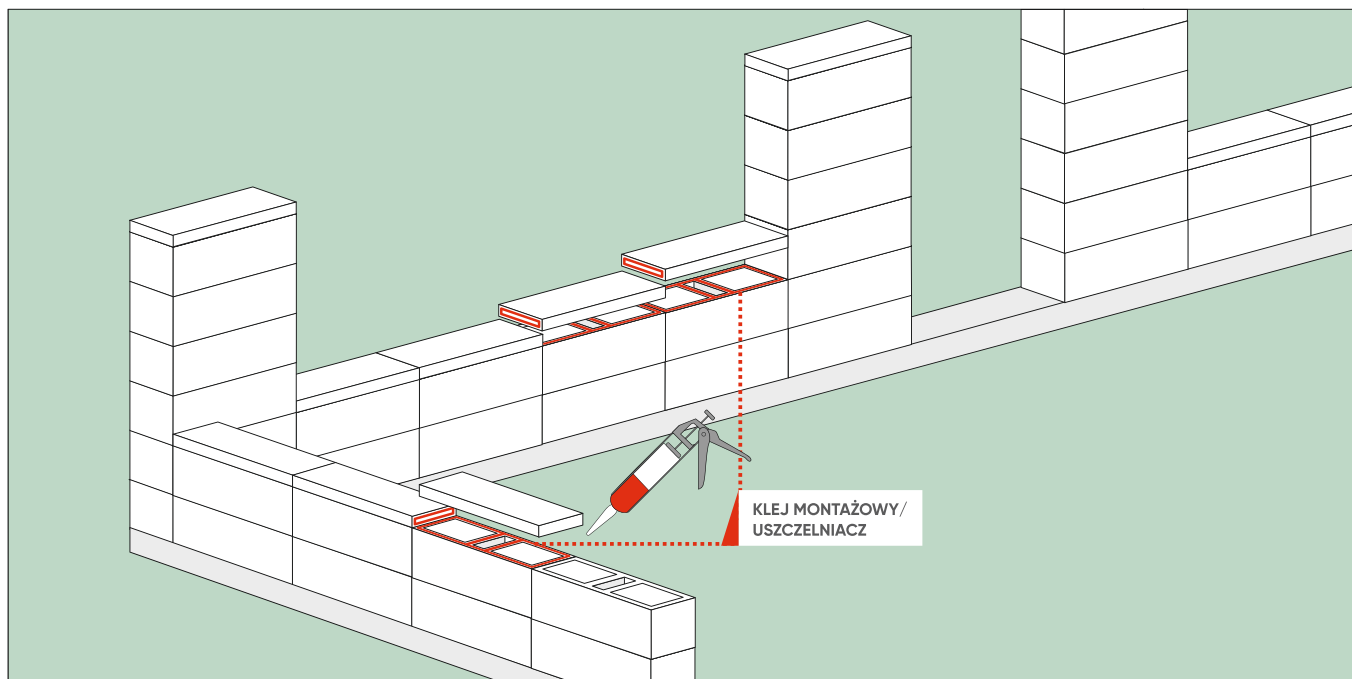
montaż daszków
