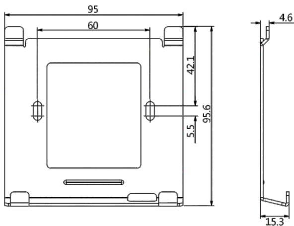
Wymiary uchwyty do montażu ściennego (M2020)
