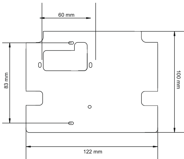
Wymiary uchwyty do montażu ściennego (M2010)
