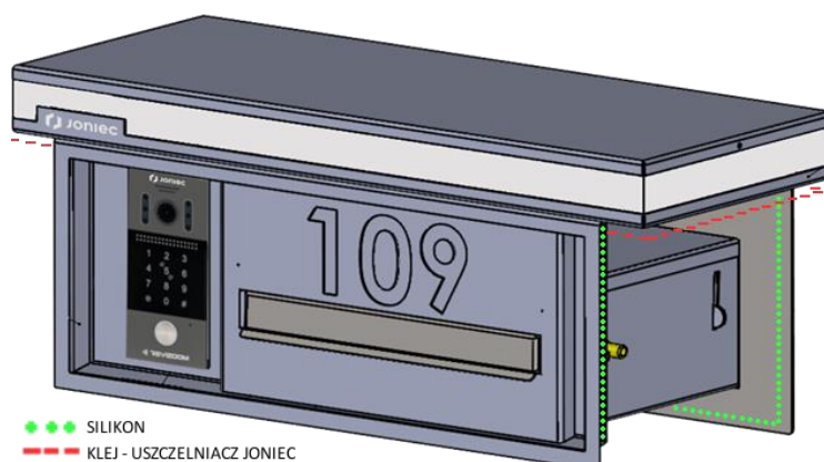
Rys 1. – schemat nakładania silikonu oraz kleju
