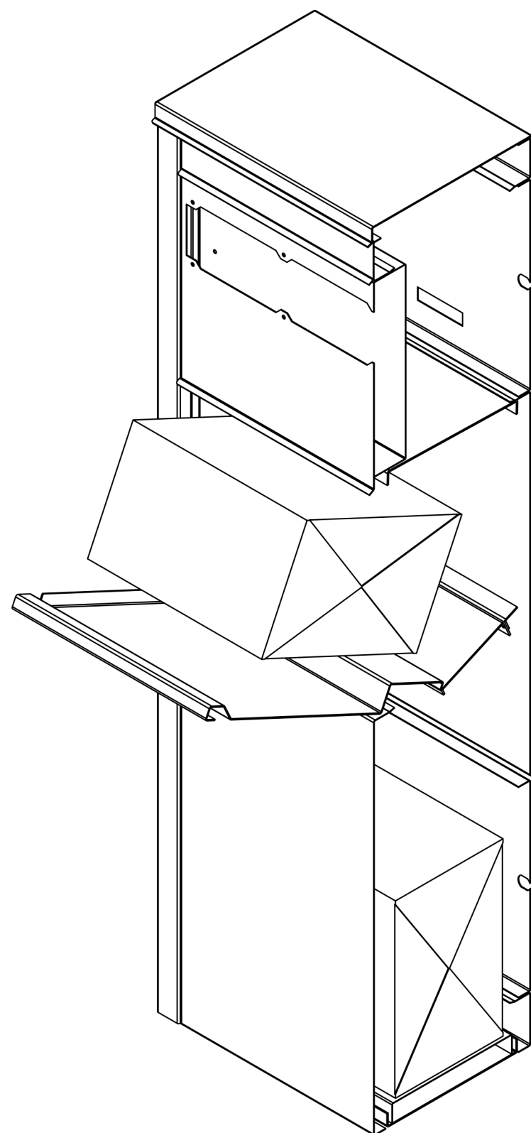
SBOX PRZEKROJ - IZOMETRIA WIZUALIZACJA WRZUTU PACZEK
