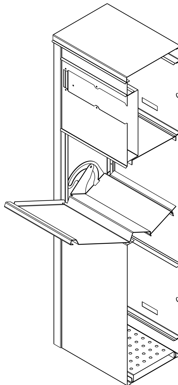
SBOX PRZEKRÓJ - IZOMETRIA
